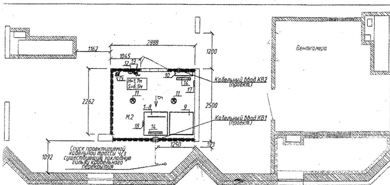
План технического этажа секции 3
