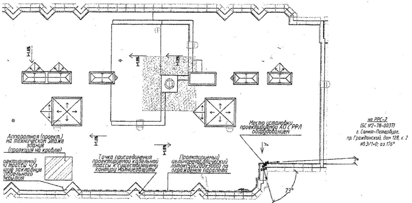
План кровли секции 3
